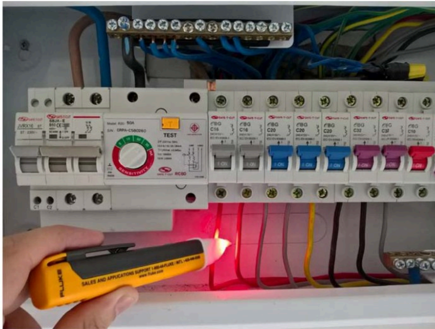
รูปที่ 101 ตรวจเช็คการติดตั้งสาย Line จาก Breaker ย่อย ถูกต้อง
