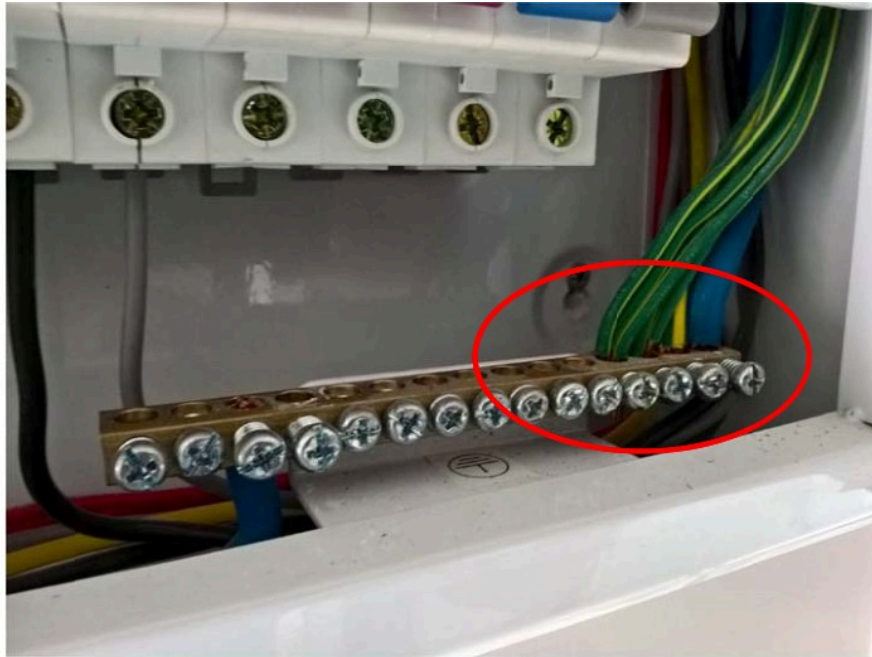
รูปที่ 99 การเชื่อมต่อสายดิน (Ground Line) ต้องไม่รวมกันเช่นนี้ (รายการแก้ไข)
